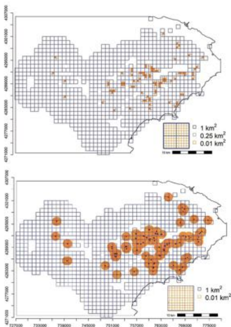
Figura 6. Representación geográfica de la intensidad de inspección en la estrategia secuencial adaptativa (arriba) y según la estrategia de vigilancia actual (Decisión 2015/789/EU) (abajo) en la zona demarcada de Alicante.
