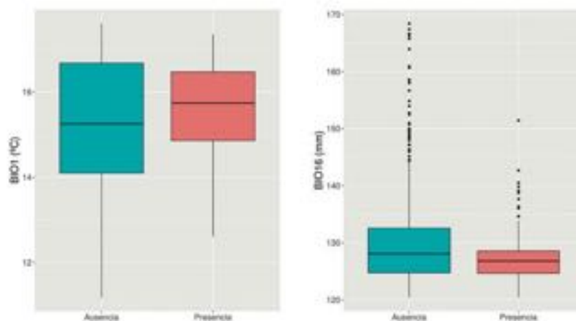
Figura 3. Representación gráfica de la temperatura media anual (BIO1) y la precipitación del mes más lluvioso (BIO16) para las cuadrículas negativas (ausencia) y positivas (presencia) para Xylella fastidiosa en la zona demarcada de Alicante. Los gráficos indican máximo, mínimo, mediana y rango intercuartílico.
