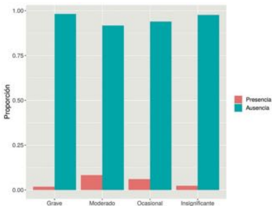
Figura 4. Proporción de cuadrículas positivas (presencia) y negativas (ausencia) para Xylella fastidiosa en la zona demarcada de Alicante para las cuatro categorías de Purcell basadas en la temperatura mínima invernal (Anas y col., 2008).
