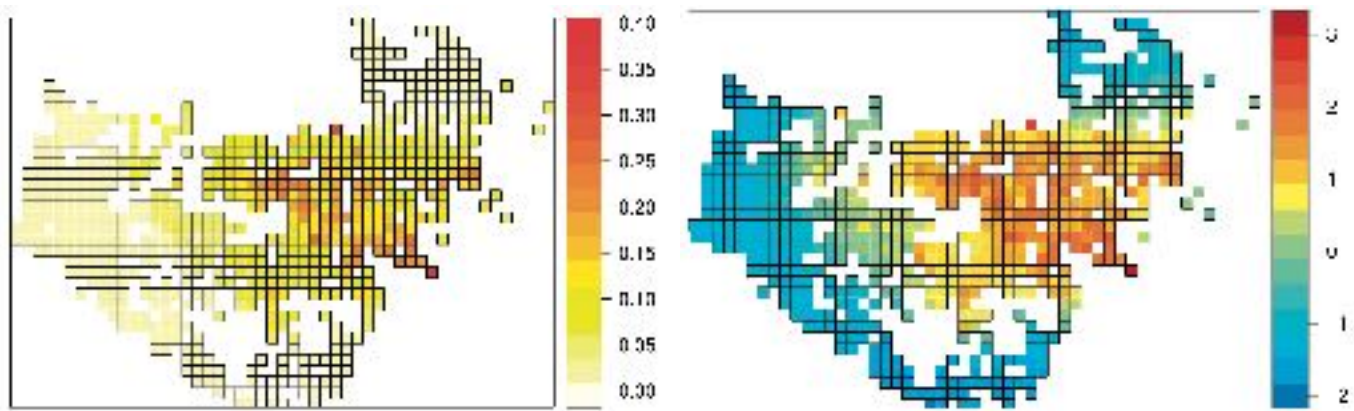
Figura 5. Modelo de la distribución geográfica de Xylella fastidiosa en la zona demarcada de Alicante. Probabilidad de presencia de X. fastidiosa , media de la distribución posterior predictiva (izquierda). Magnitud del efecto espacial, media de la distribución posterior del efecto espacial (derecha).
